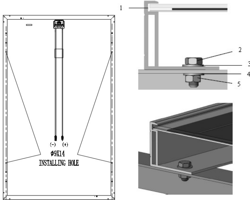
图 7 光伏组件的螺栓安装方式
